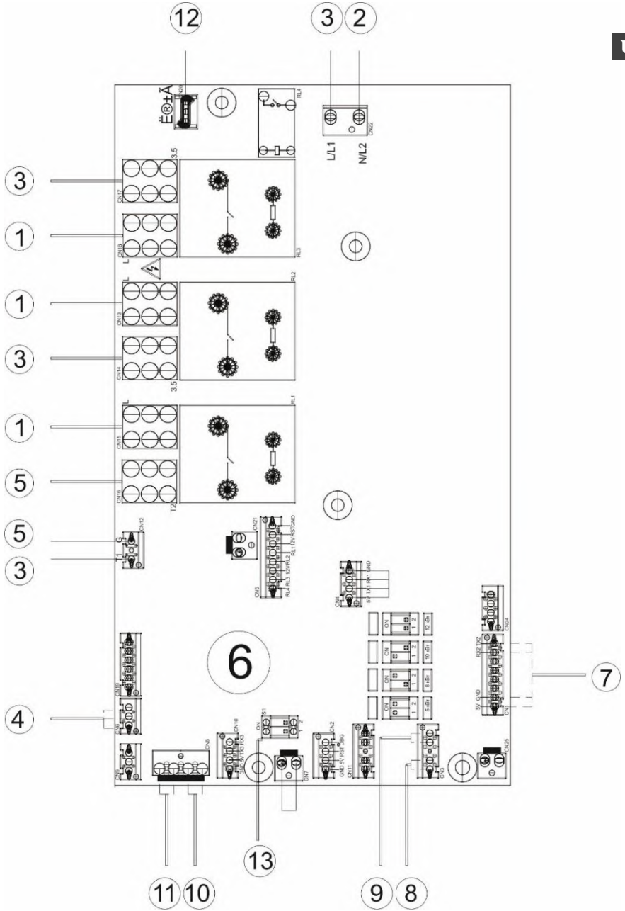
Мал. 16. Електрична схема основної плати керування
