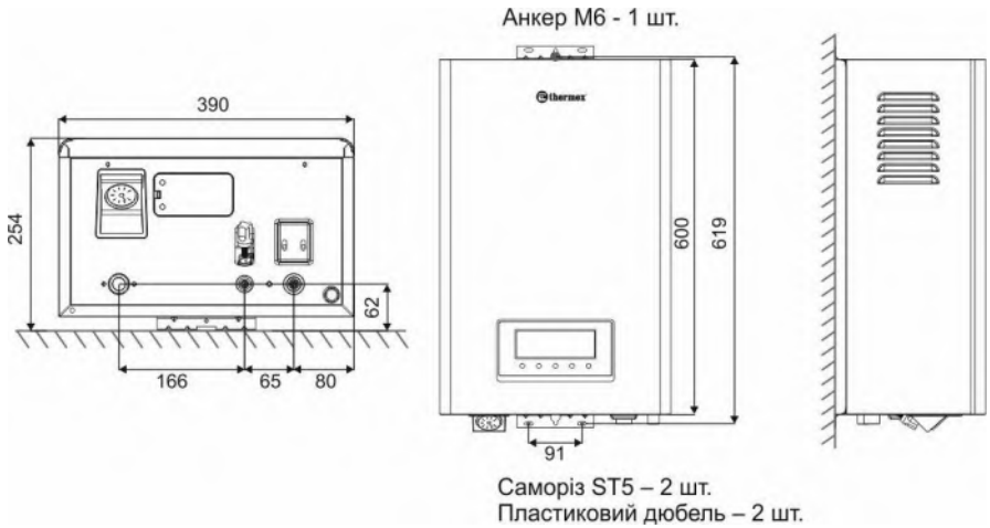
Мал. 6. Монтажні розміри
