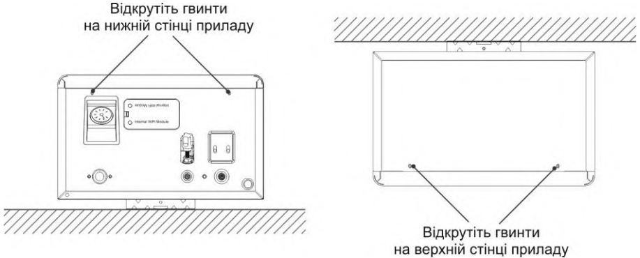
Мал. 8. Демонтаж лицевої панелі
