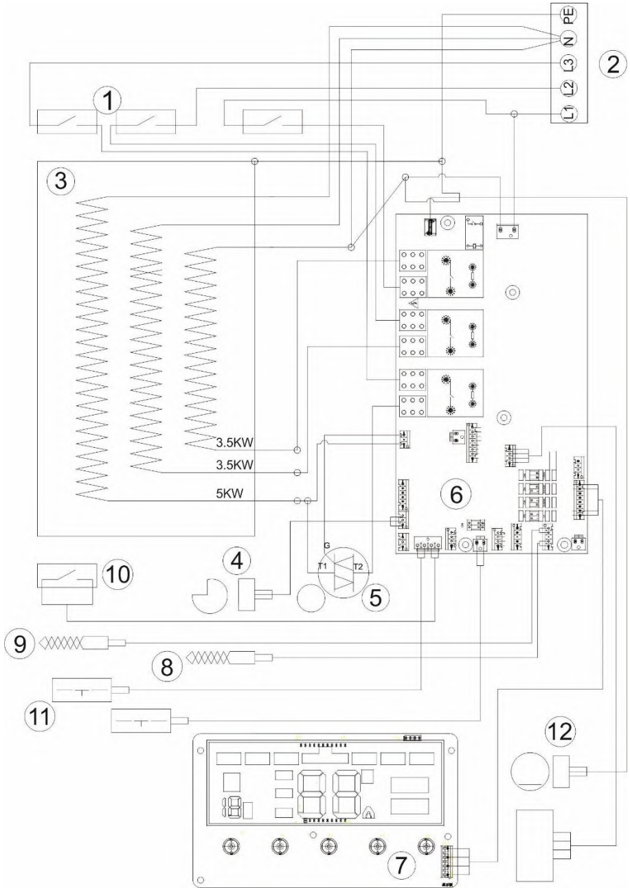
Мал. 15. Електрична схема THERMEX Grizzly 5-12 Wi-Fi
