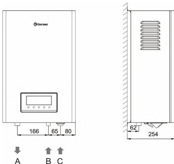
Мал. 7. З'єднувальні розміри
